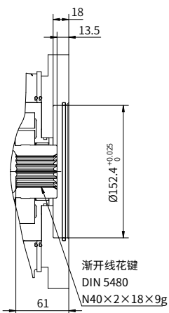
“D4”型通轴驱动
