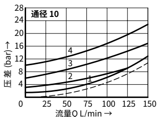
\Delta P -Q 曲线 - 底板连接
