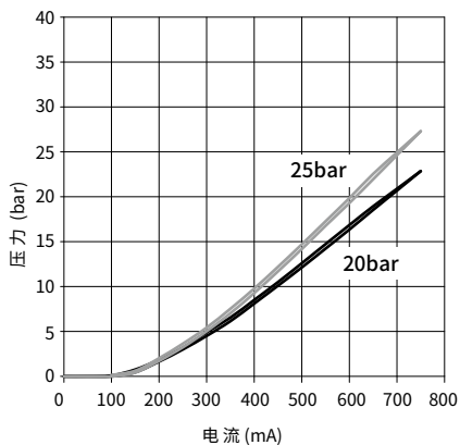
P-I 曲线 (24V)
