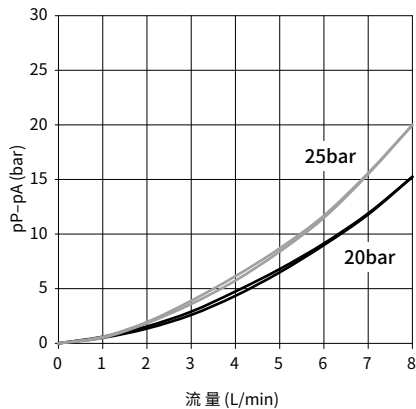
压力损失 (P→A)
