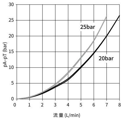
压力损失 (A→T)
