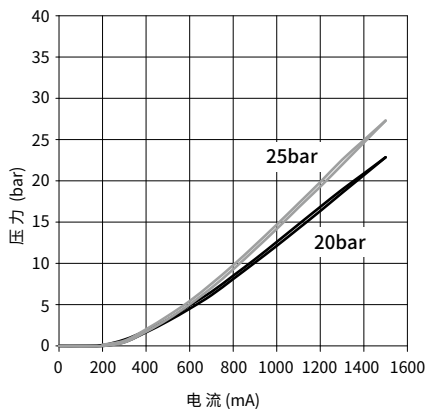
P-I 曲线 (12V)
